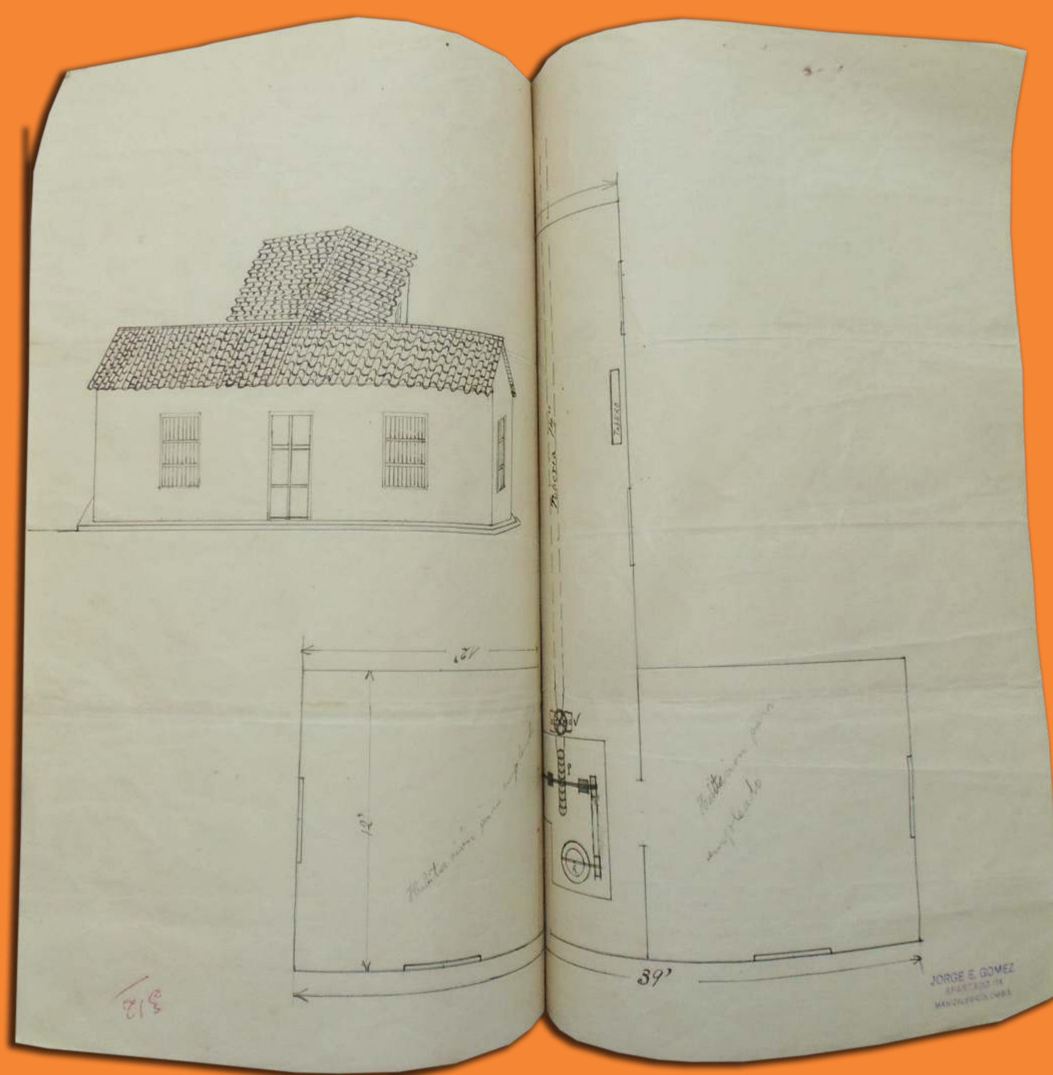
Plano de la planta hidroeléctrica de Salento con habitaciones para empleados. Cerca a 1929.
